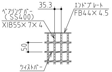
グレーチング構造図
